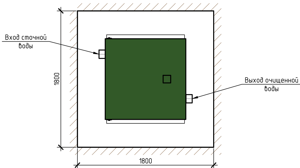
Вид сверху
