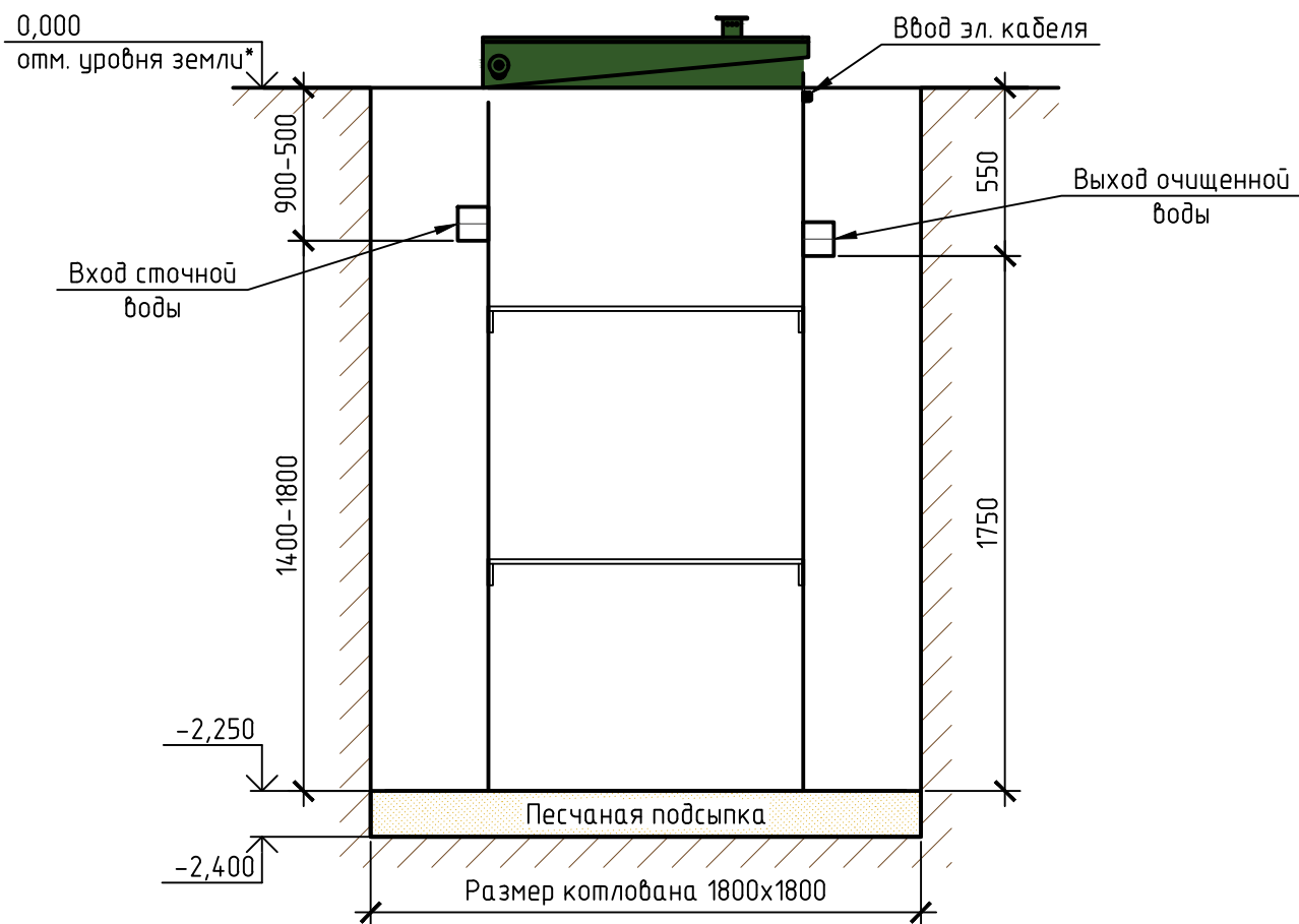
Вид сбоку
